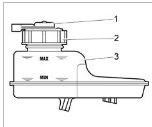
Рис. 46. Бачок гидропривода тормозов
