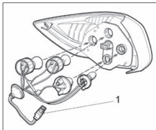
Рис. 57б. Задний фонарь автомобиля с кузовом «лифтбек»
