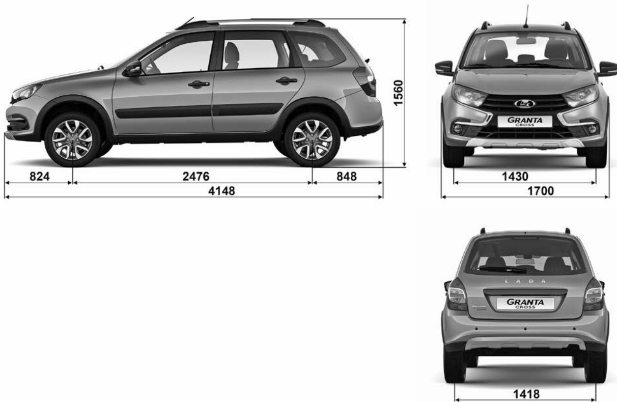
Рис. 62д. Габаритные (справочные) размеры автомобиля в модификации «Cross»
