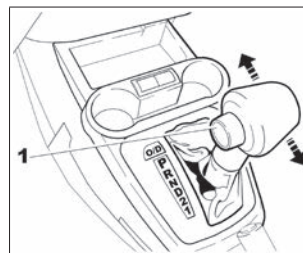
Рис. 36а. Рычаг переключения передач в автоматической коробке передач
