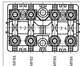
Рис. 55б. Блок предохранителей моторного отсека
