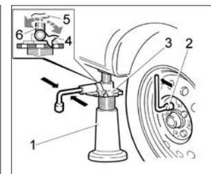
Рис. 50б. Подъем автомобиля при замене колес
