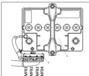
Рис. 55а. Блок предохранителей моторного отсека
