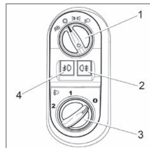
Рис. 30. Модуль управления светотехникой и корректор ближнего света фар
