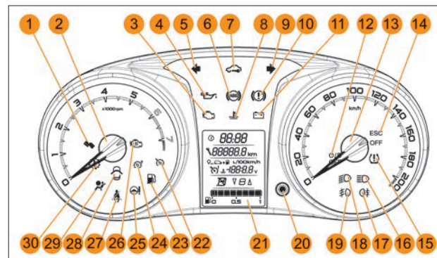
Рис. 29а. Комбинация приборов
