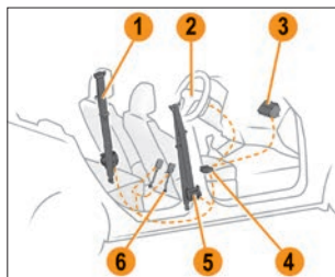
Схема устройства системы пассивной безопасности (в варианном исполнении)
