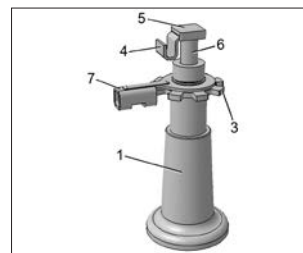
Рис. 50в. Домкрат (в варианном исполнении)
