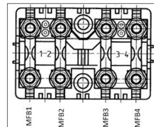
Рис. 55б. Блок предохранителей моторного отсека
