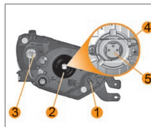
Рис. 56. Блок-фара
