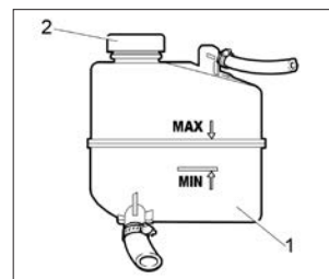
Рис. 45. Расширительный бачок
