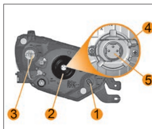
Рис. 56. Блок-фара
