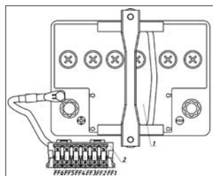
Рис. 55. Блок предохранителей моторного отсека
