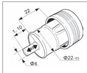
Рис. 21в. Размеры вилки электрического прибора для использования в патроне для подключения дополнительных потребителей
