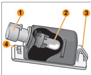
Рис. 58а. Фонарь освещения номерного знака
