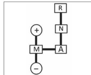
Рис. 36д. Схема переключения передач
