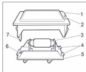
Рис. 59. Плафон освещения багажника автомобиля с кузовом «седан»
