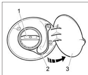
Рис. 27. Пробка топливного бака
