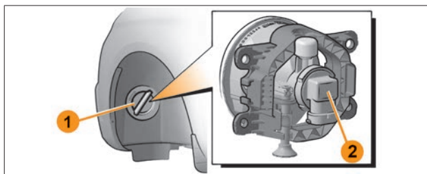
Рис. 61. Противотуманная фара
