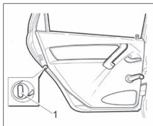
Рис. 8. Шлиц защелки
