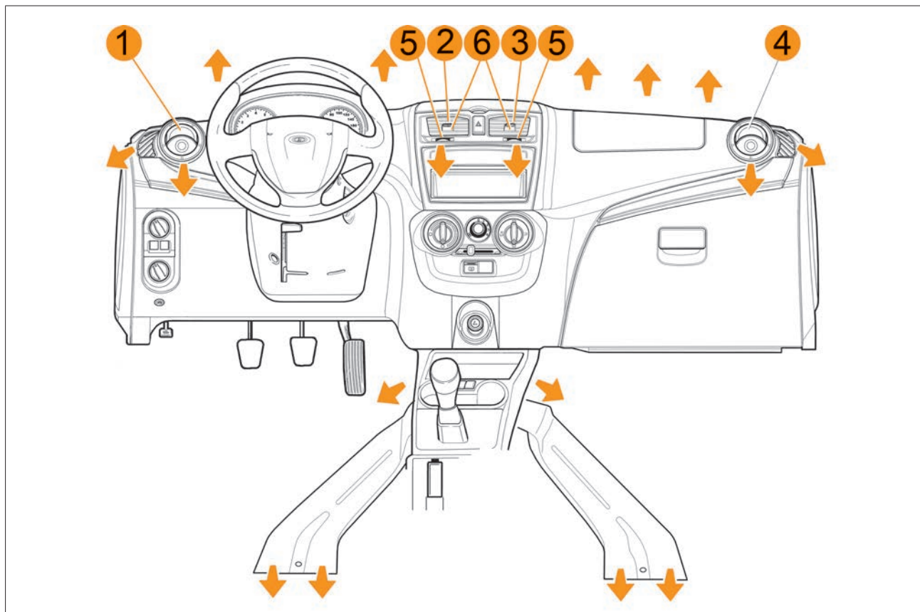
Рис. 38а. Направления потоков воздуха из дефлекторов и воздуховодов
