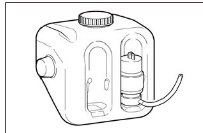
Рис. 50. Бачок омывателей ветрового стекла
