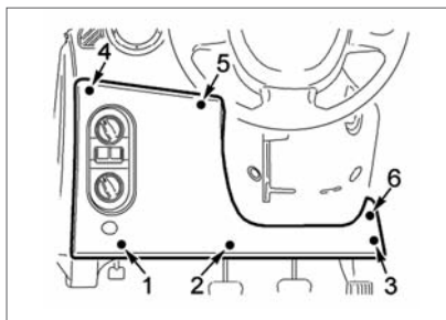
Рис. 56. Открытие крышки монтажного блока
