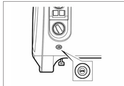
Рис. 26а. Выключатель привода замка багажника (в варианном исполнении)
