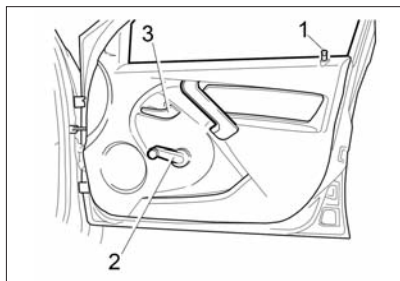
Рис. 6а. Передняя правая дверь
