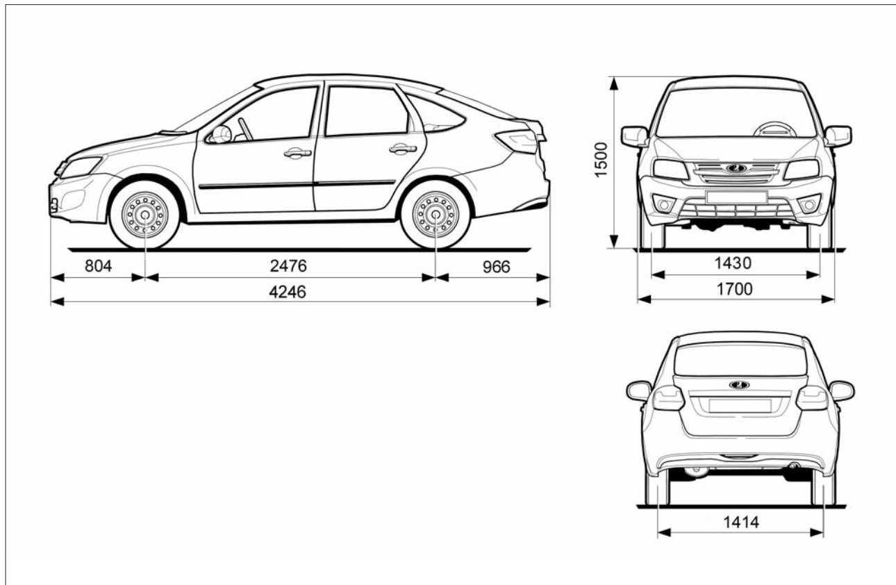
Рис. 656. Габаритные (справочные) размеры автомобиля с кузовом «лифтбек»
