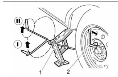
Рис. 53а. Подъем автомобиля при замене колес
