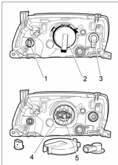
Рис. 60. Блок-фара
